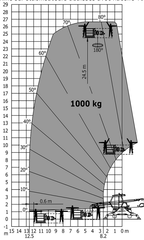
Machine sur stabilisateurs abaissés avec nacelle 1000 kg
