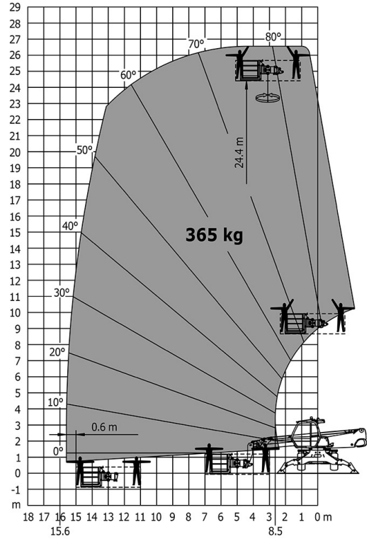
Machine sur stabilisateurs abaissés avec nacelle 365 kg
