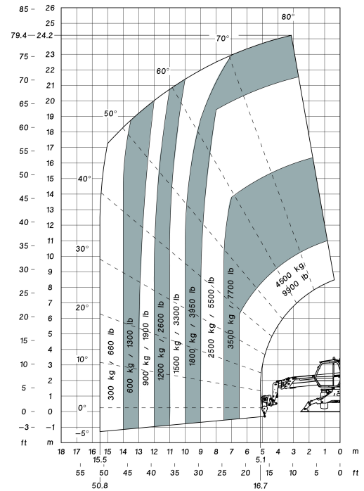
Machine sur stabilisateurs abaissés avec treuil 5000 kg
