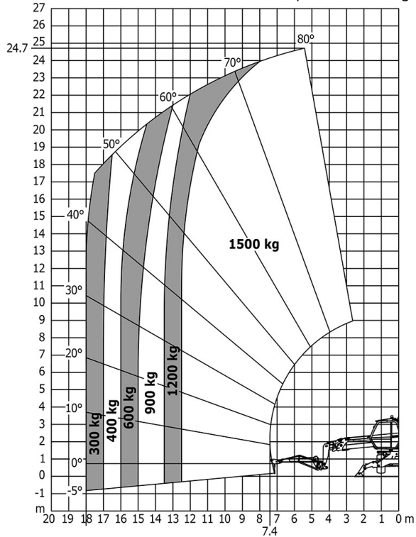
Machine sur stabilisateurs abaissés avec potence 1500 kg
