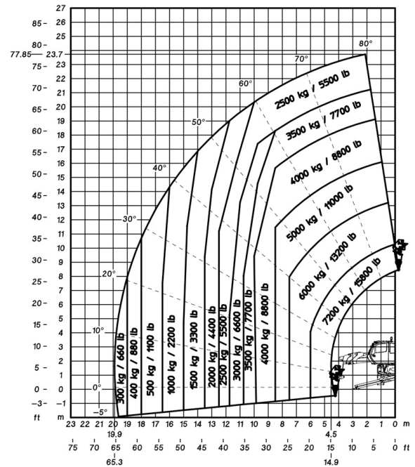
Machine sur stabilisateurs abaissés avec treuil 7200 kg (métrique)
